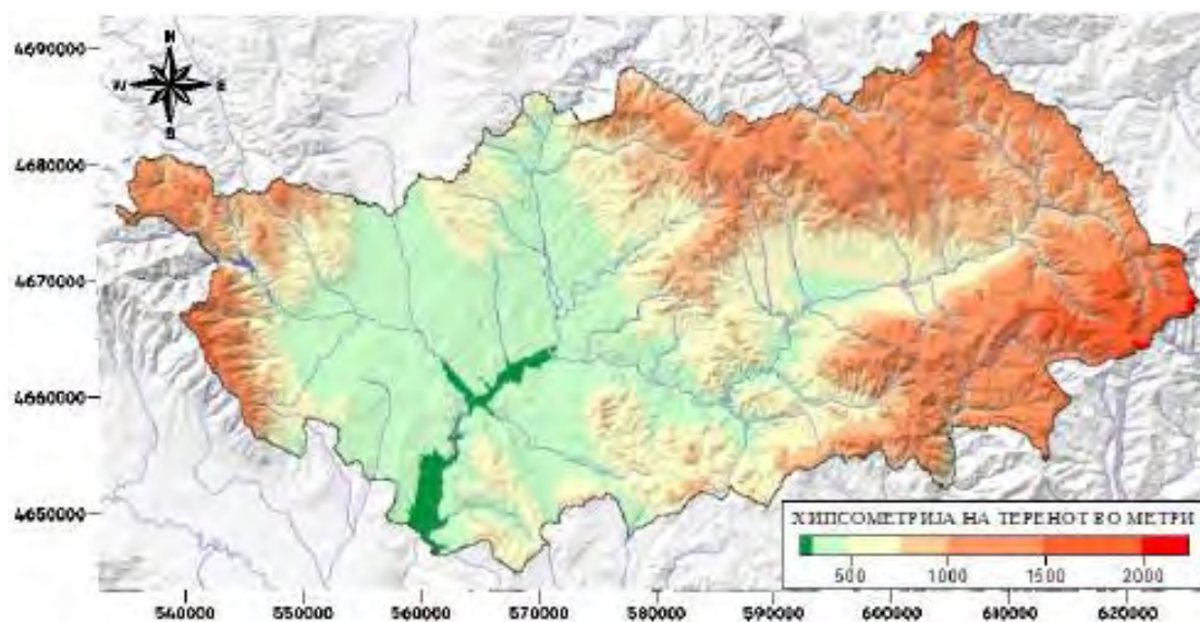
Слика 18. Релјеф на Североисточен Регион
