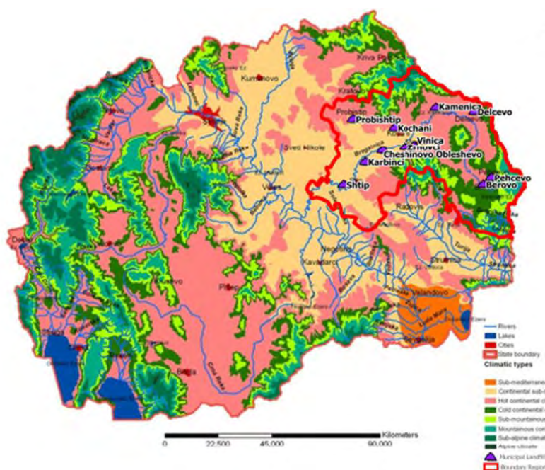
Слика 9. Климатска карта во Источен Регион
