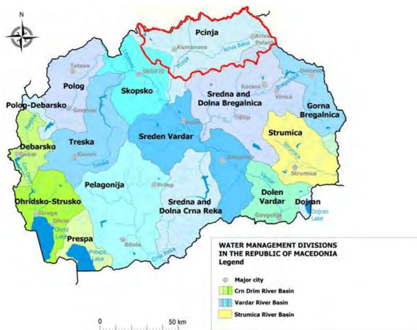
Слика 15. Речни сливови и подрачја на речни сливови во „Североисточниот“ регион, Република Северна Македонија (според Националната стратегија за води, 2011 – 2041 година)
