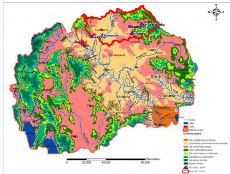
Слика 10. Климатска карта во Североисточниот Регион
