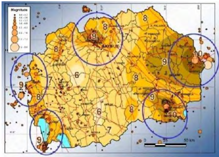
Слика 21. Сеизмичка карта на Северна Македонија
