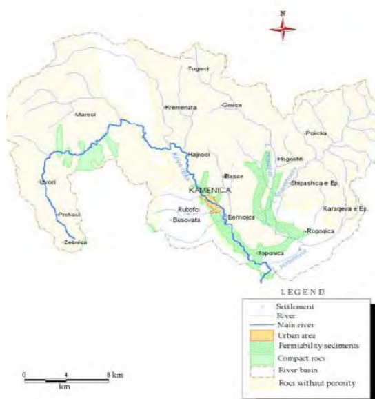
Слика 14. Хидрогеолошка карта на сливот на Крива Река (Извор: „Хидрогеографски карактеристики на Крива Река“)
