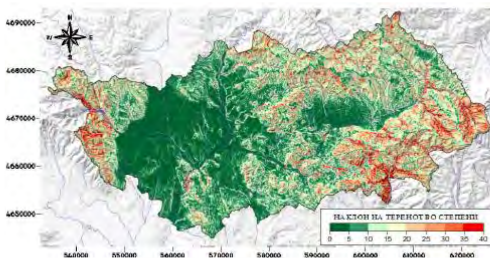
Слика 19. Релјеф на Североисточен Регион
