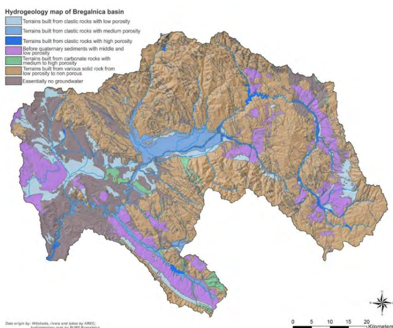
Слика 11. Хидрогеолошка карта на сливот на реката Брегалница
