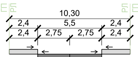
станбена улица ул. "5-та Партиска Конгеренција" ПРОФИЛ 3-3
