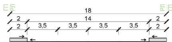
собрна улица по ГУП ул. "Сремски Фронт" ПРОФИЛ 1-1
