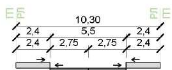
станбена улица ул. "5-та Партиска Конгеренција" ПРОФИЛ 3-3
