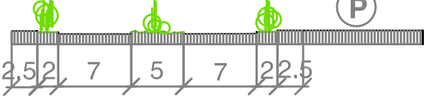
ПРОФИЛ НА МАГИСТРАЛНА УЛИЦА "ГОЦЕ ДЕЛЧЕВ" - пресек 2 - 2
