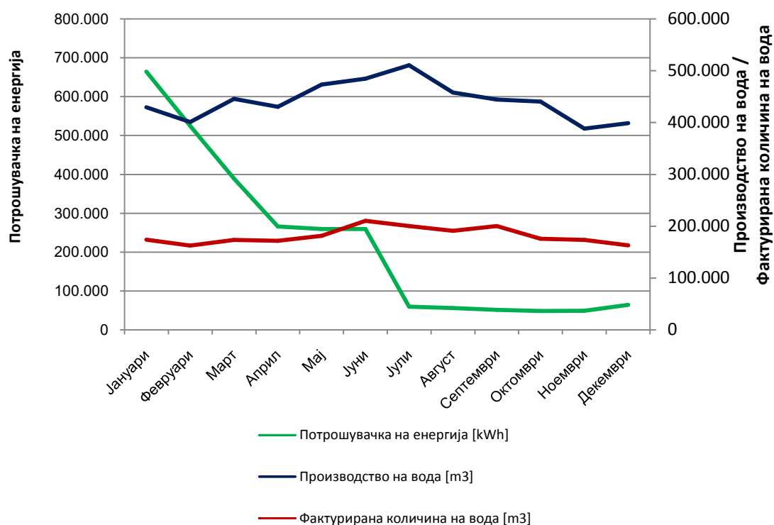
Слика 4: Потрошувачка на електрична енергија, производство на вода и фактурирана количина на вода за референтната година 2022 (пример)
