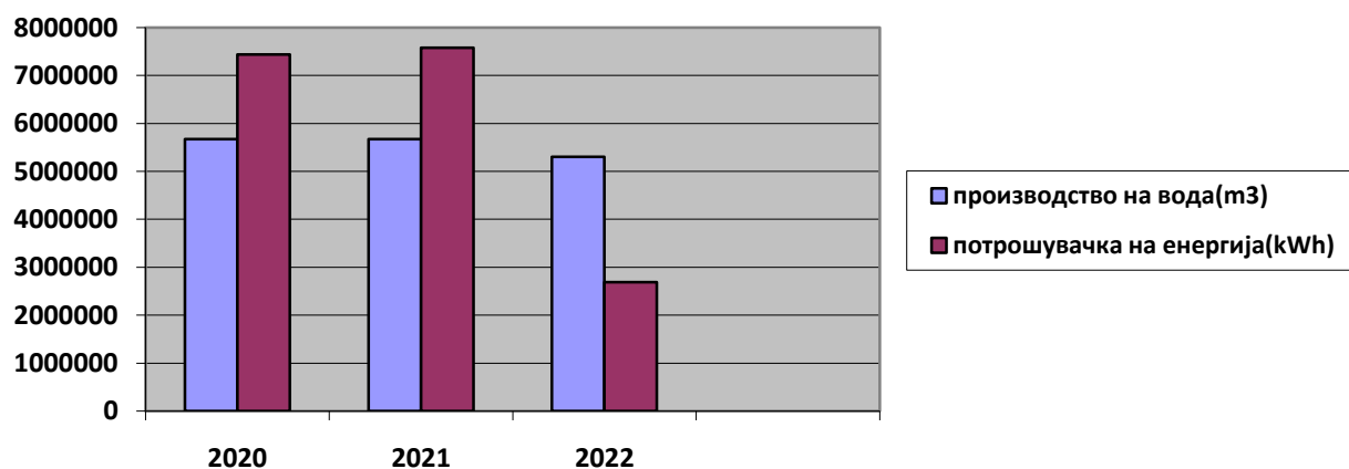
Слика 3: Производство на вода и потрошувачка на електрична енергија во периодот од 2020 – 2022
