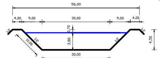
Слика: Попречен пресек на коритото на реката Брегалница кај Штип (вонградски дел) P=1:100/200
