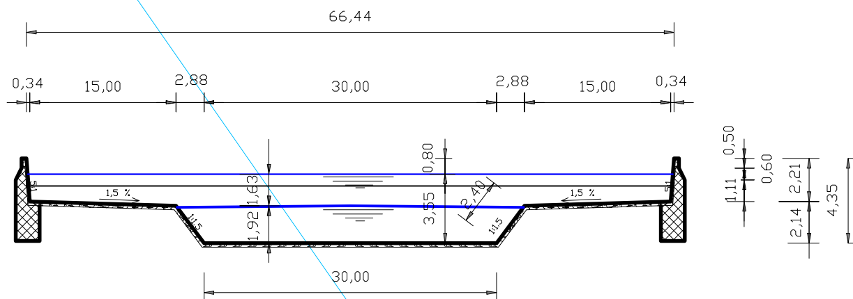
Слика: Попречен пресек на коритото на реката Брегалница кај Штип (градски дел) P=1:100/200
