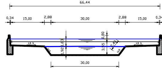
Слика: Попречен пресек на коритото на реката Брегалница кај Штип (градски дел) P=1:100/200
