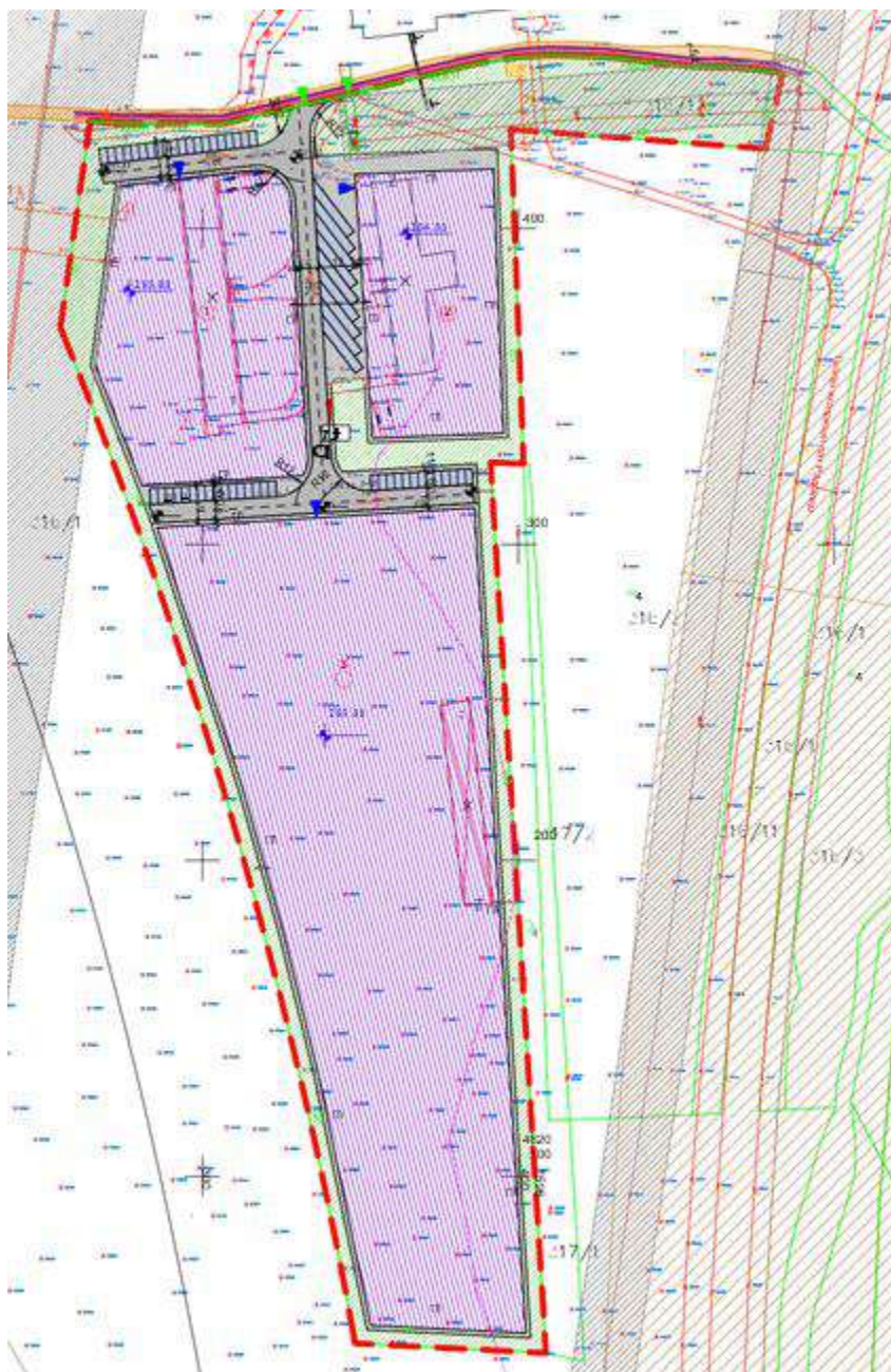
Графички приказ на Урбанистички проект вон опфат на урбанистички план Г-4 Стоваришта, складови и отпади на дел од КП 316/1, КО Ново Село Штип, општина Штип
