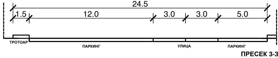
ПРОФИЛ НА УЛИЦА 2 ВО ПАРЦЕЛА
