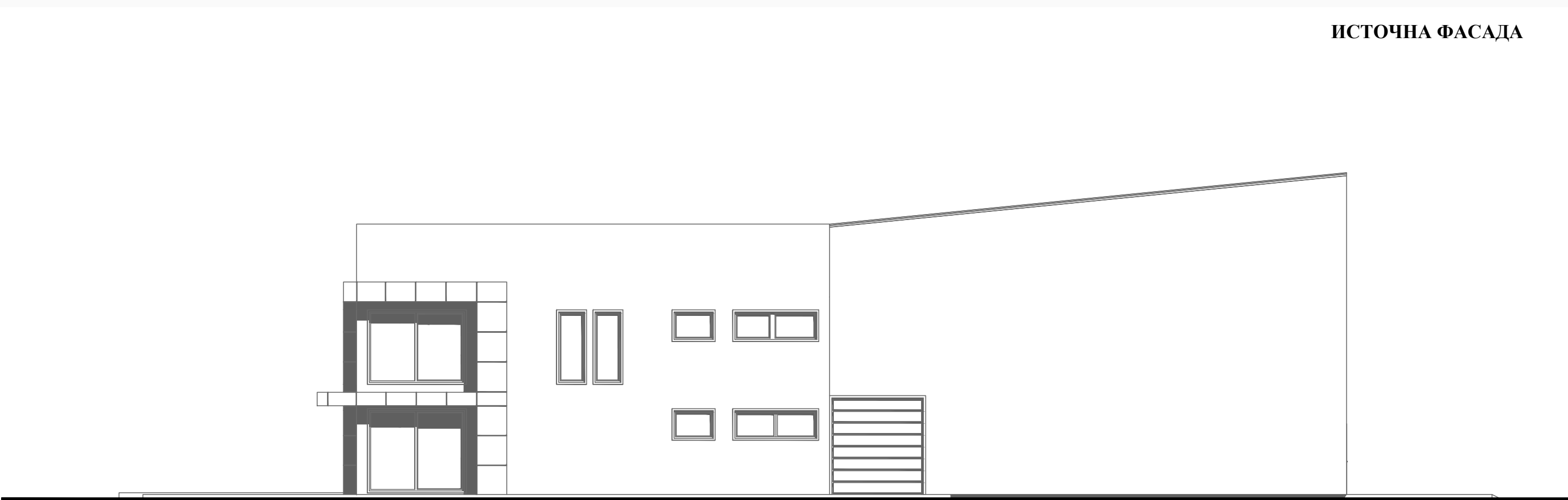
СЕВЕРНА ФАСАДА
