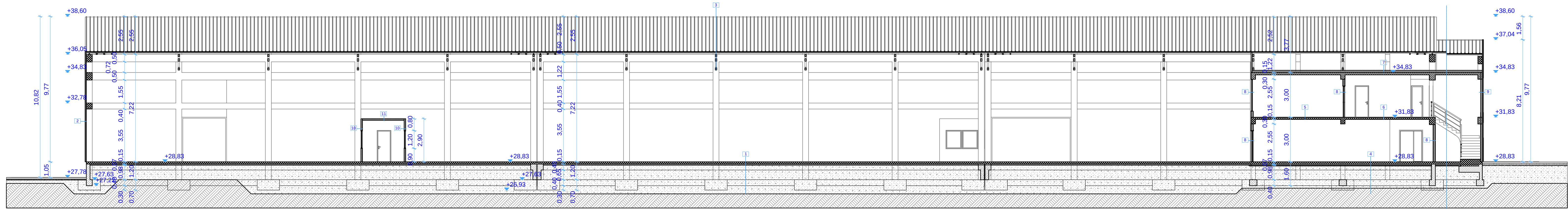
ПРЕСЕК 1-1 1:100
