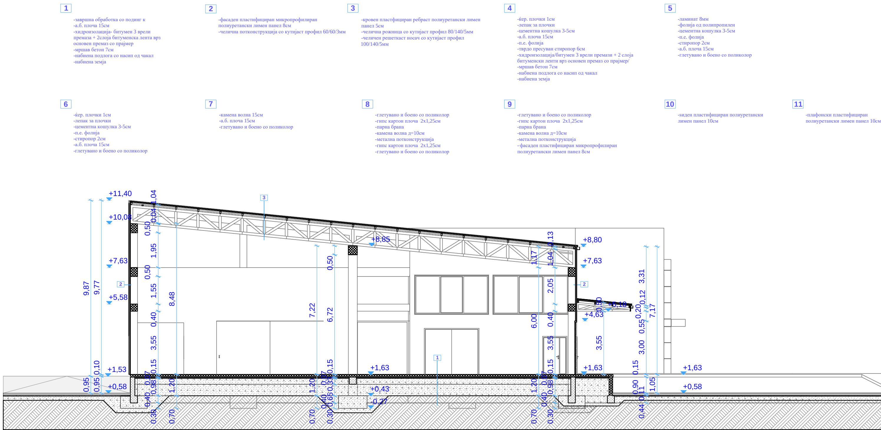
ПРЕСЕК 2-2 1:100
