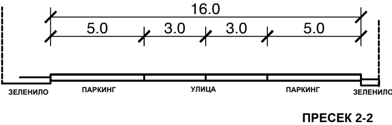
ПРЕСЕК 2-2
